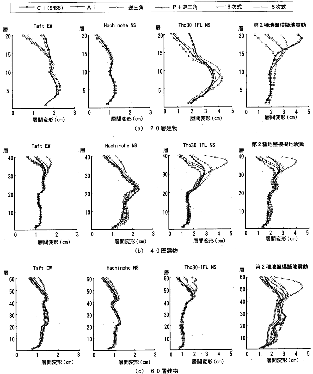
図-6 設計用せん断力係数分布の違いによる最大応答層間変形の相違
