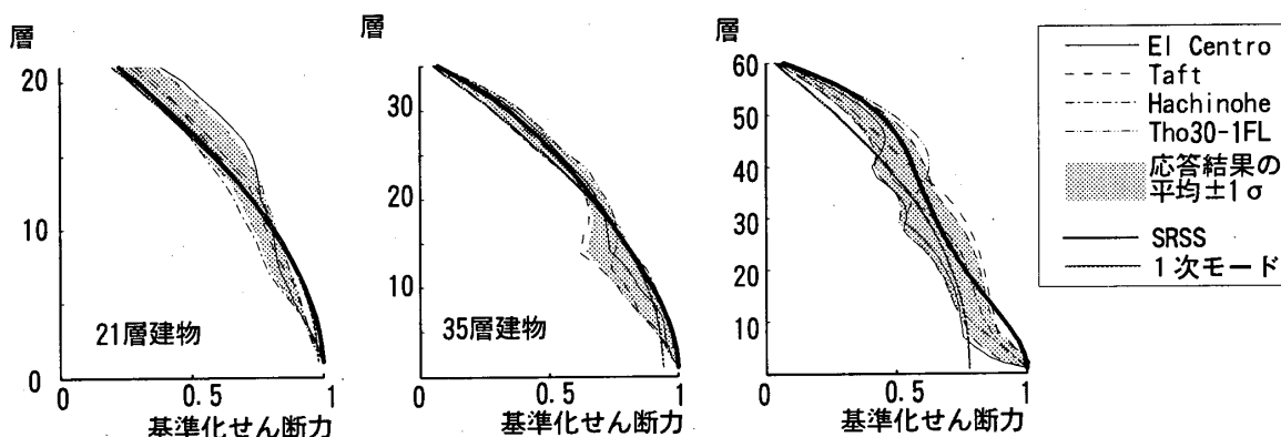
図-4 規準化した応答せん断力分布
