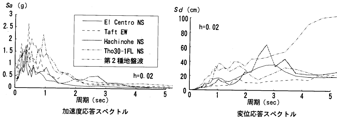
図-1 使用した地震動記録の応答スペクトル
