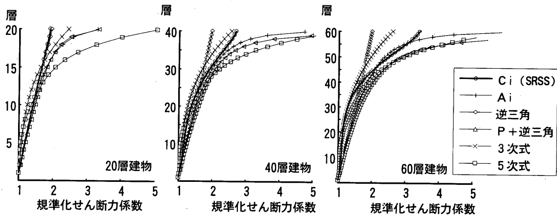
図-5 各種せん断力分布の比較
