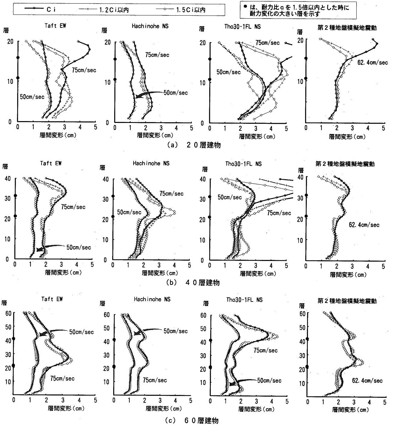
図-10 耐力比の違いによる最大応答層間変形の相違 (図中の数字は入力地震動の最大速度振幅を示す)
