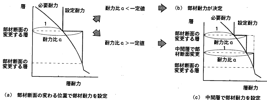
図-8 部材耐力の設定法
