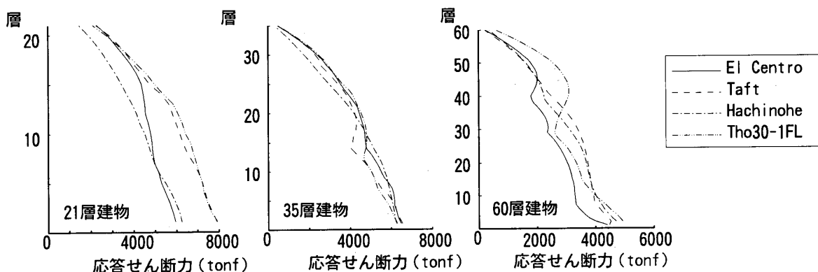
図-3 応答せん断力の分布
